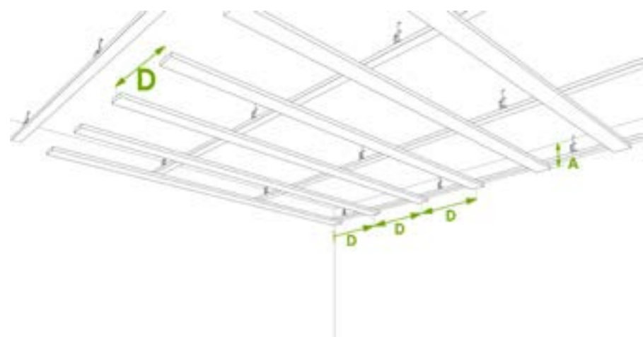
Abb. 2b Zweite Unterkonstruktion mit Holzlatte Achsabstand D= 600mm (zwingend erforderlich!)
